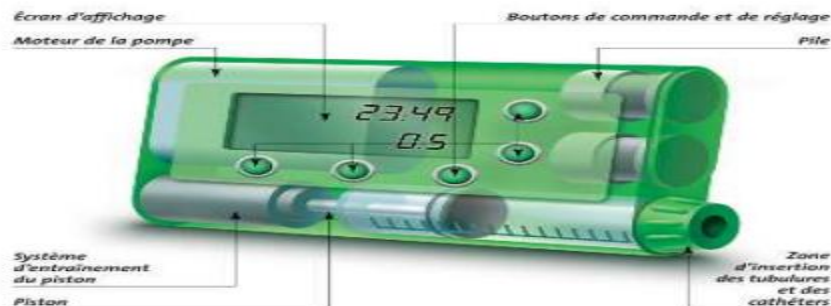
Figure 3 : Détail des Composants de la Pompe
